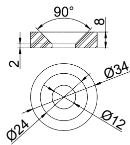
Washer(1 no- MS)
