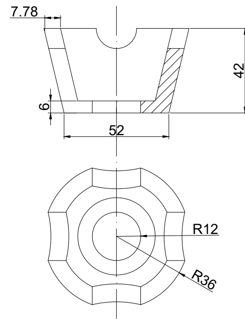
Cup(1 no- CS)
