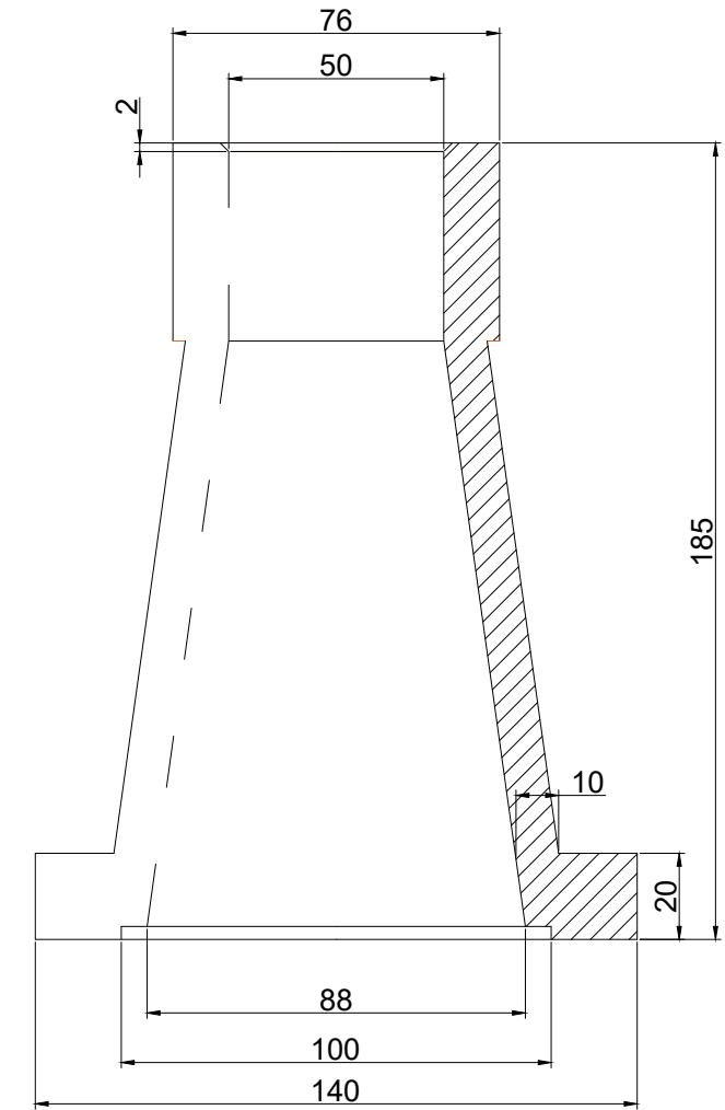
Body (I No -CI)
