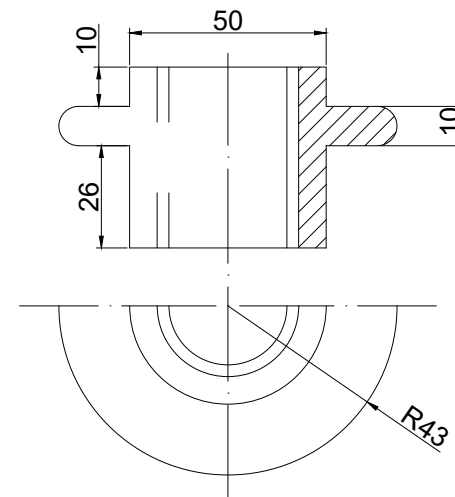
Nut (1 No - G.M)
